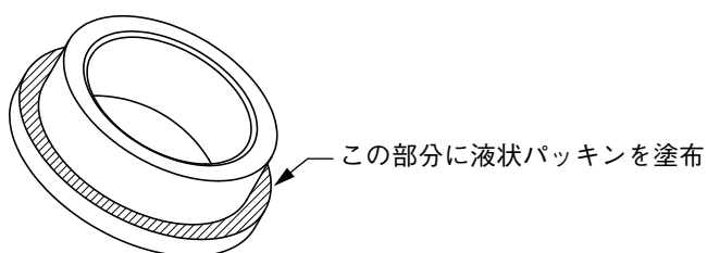
図 3-7 シートリンク
