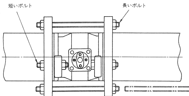
図 2-2 配管への取り付け
