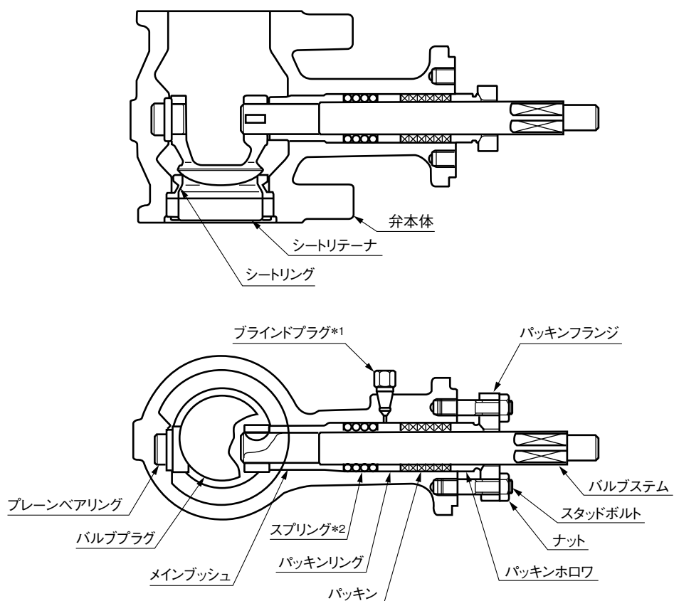
図 3-2 断面図
