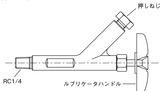
図 2-3 ルブリケーター
