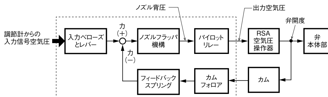
図 5-5 ポジショナのブロック線図
