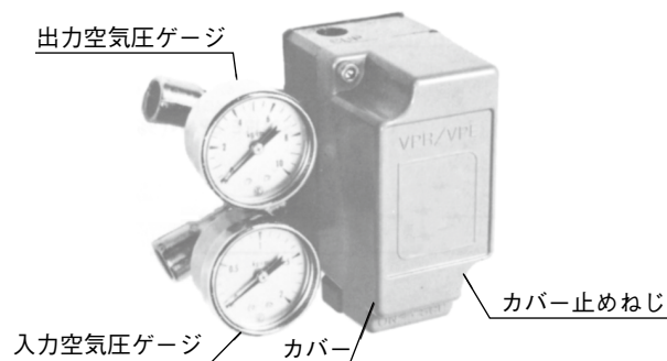
図 5-4 正面
