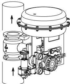
図B-4 配管取付姿勢(AVP 電/空ポジショナ+減圧弁一体)
