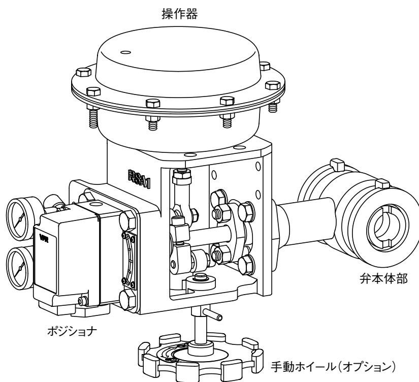
図 1-1 VFR 調節弁の構成
