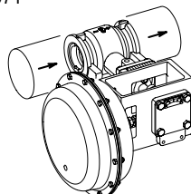
図B-3 配管取付姿勢(ポジションなし)
