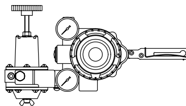
AVP(減圧弁一体形)
