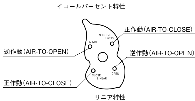
図 5-13 カム
