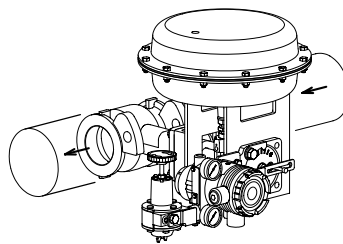
図B-4 配管取付姿勢(AVP 電/空ポジショナ+減圧弁一体)
