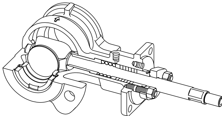
図 3-1 構造図
