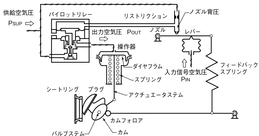
図 5-6 動作原理図
