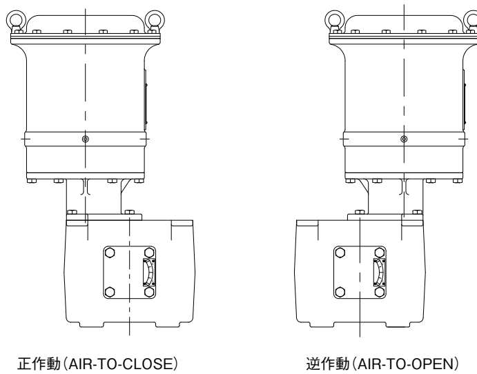
図 5-12 操作器作動
