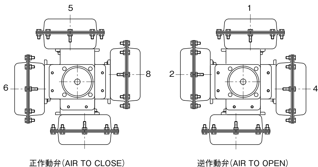
図 6-1 取付姿勢
