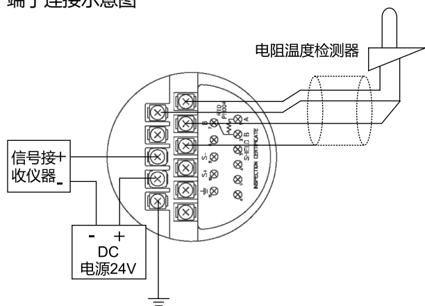
端子连接示意图
