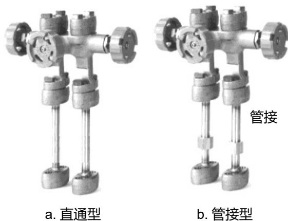
图 2-4 延长管
