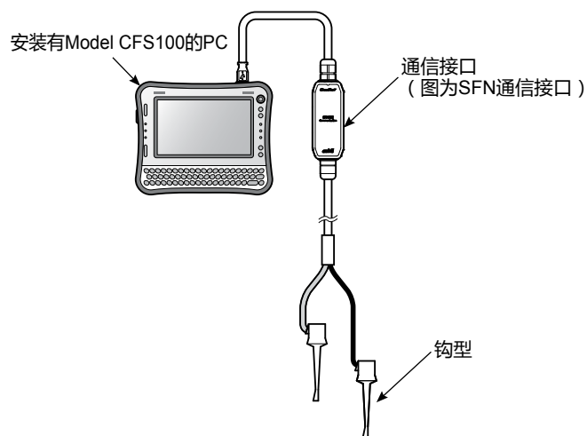
图 1-7 Model CFS100 的构成
