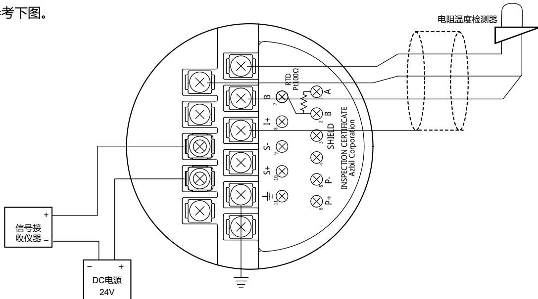
图 2 - 9 配线、接地端子示意图
