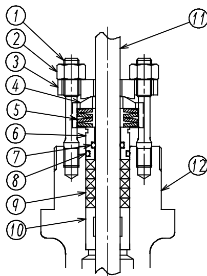
図 8-1 SECURE-SEAL 構成図
