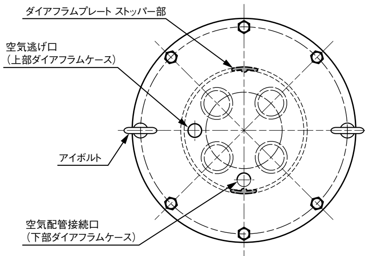
図 6-11 逆作動 (PSA1R)
