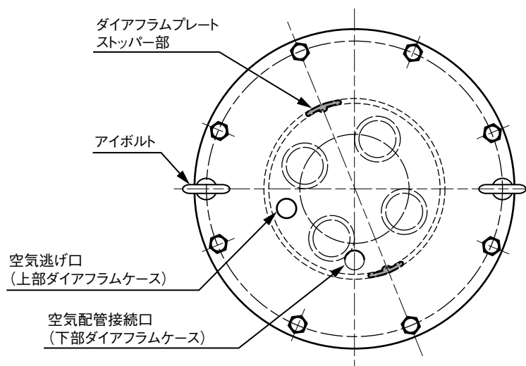
図 6-12 逆作動 (PSA2R)
