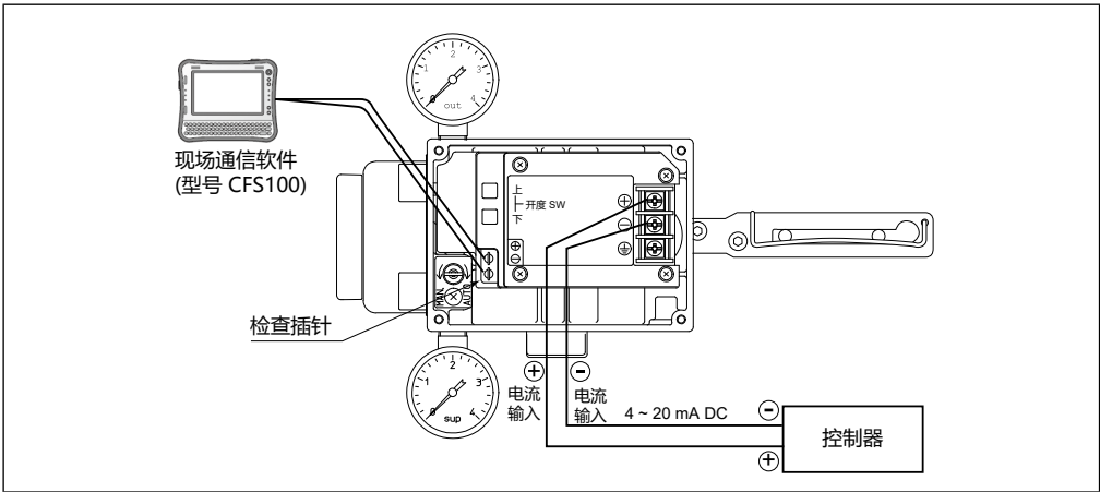
图 4-2. 带现场通信软件 (AVP100/102 型) 的布线
