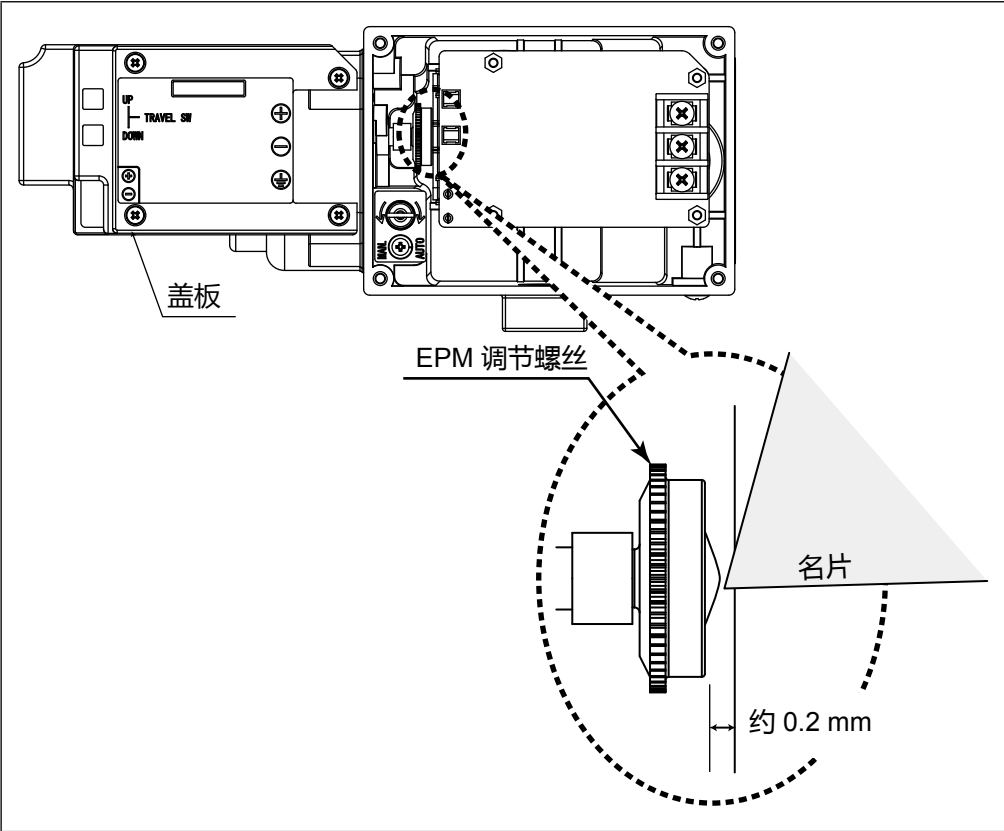
图 5-5. EPM 平衡调整
