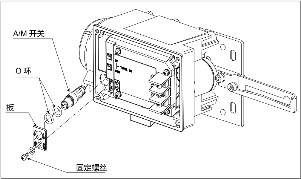
图 5-4. A/M 开关
