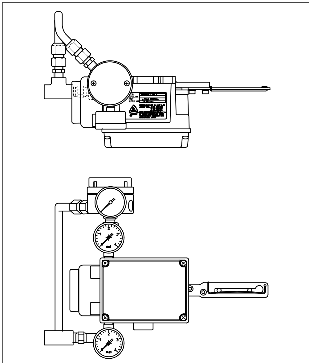
图 2-11. 未直接连接空气调节器的双作用 SVP
