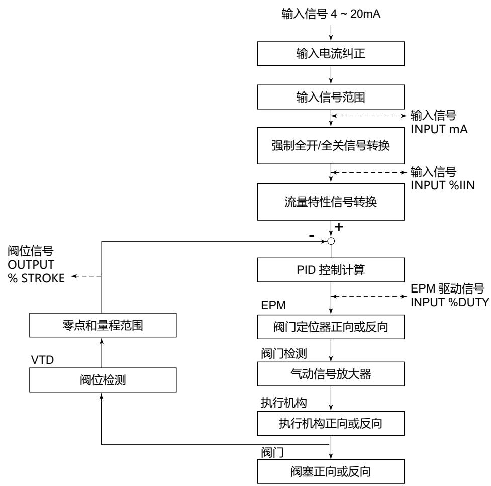
图 5-8. SVP I/O 流程图
