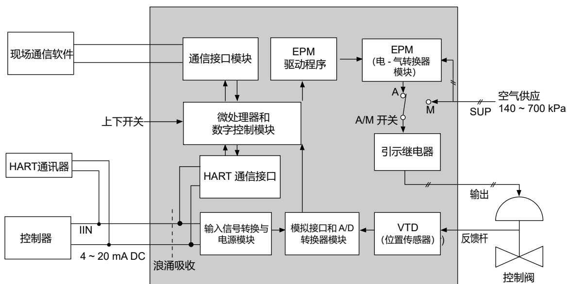
图 5-7. SVP 方块图
