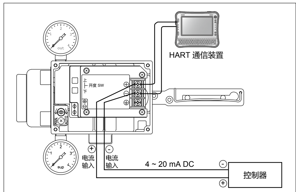
图 1-2. HART 通信结构
