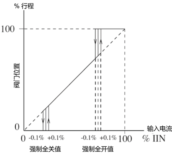
图 4-4. 强制全开/全关设定
