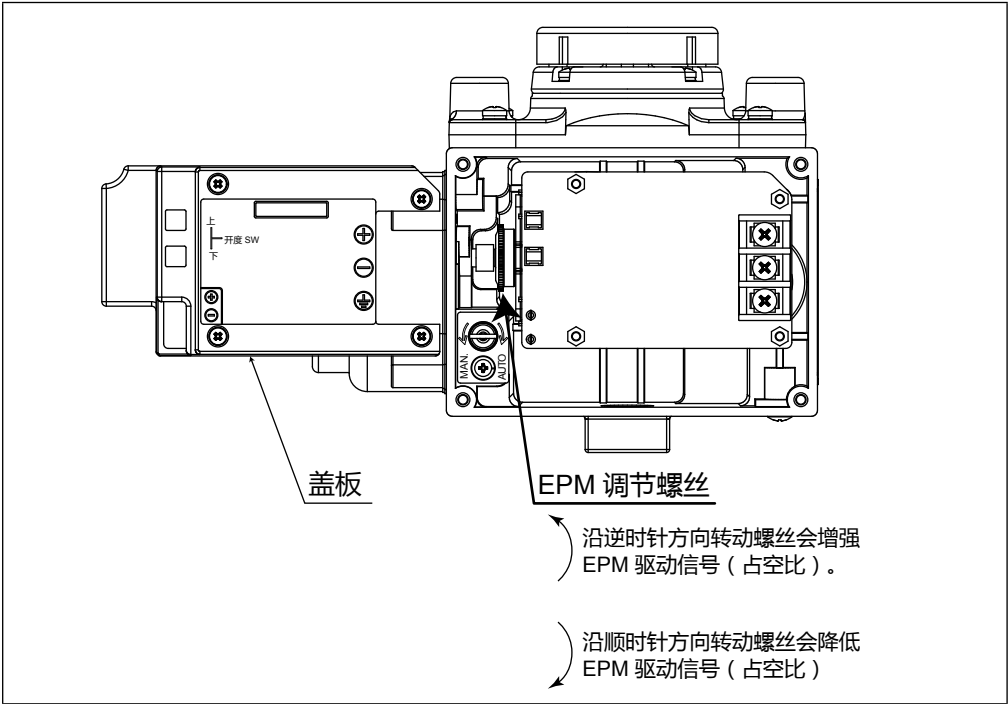
图 5-6. EPM 平衡调整
