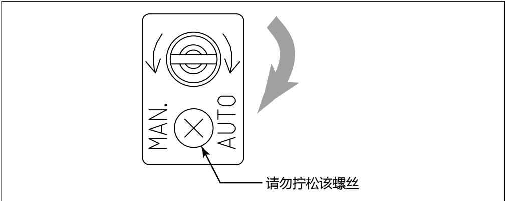
图 5-3. 从手动操作状态切换到自动操作状态
