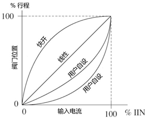
图 4-3. 流量特性概述
