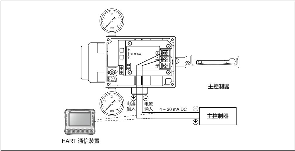
图 4-1. HART® 通信工具 (AVP102 型) 的布线
