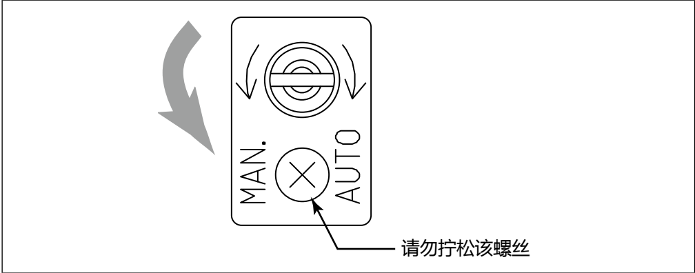
图 5-2. 从自动（正常）操作状态切换到手动操作状态
