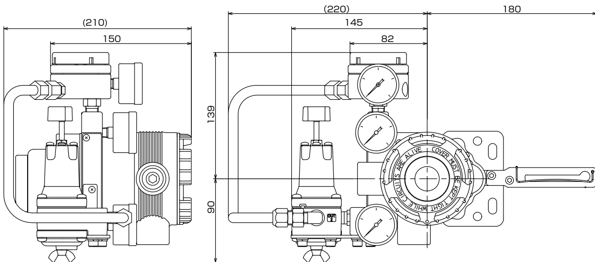
<複動用リバーシングリレー付、形 RA1B 減圧弁付>
