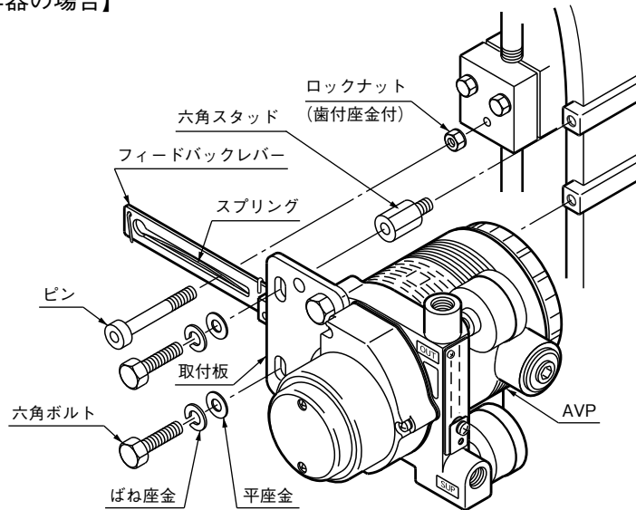
図 2-1-1 AVP の HA1 操作器への取付方法
