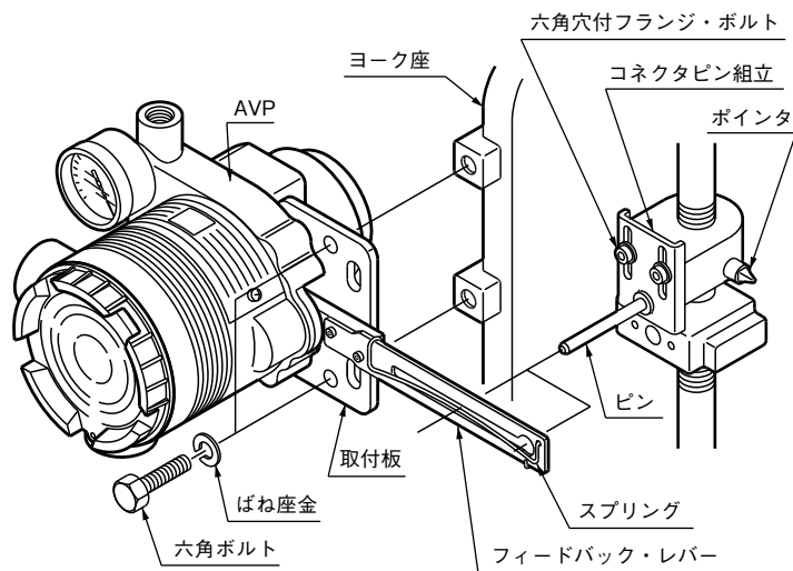
図 2-1-2 AVP の HA2、3、4、PSA1～4、6、VA1～6 操作器への取付方法
