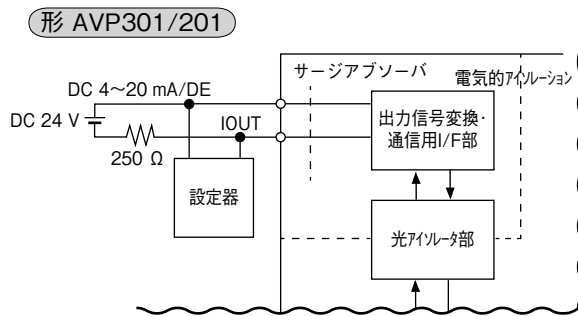
図 5-2 内部ブロック図
