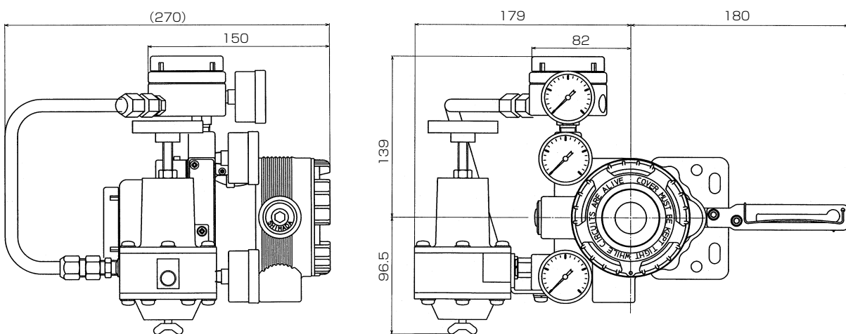
<複動用リバーシングリレー付、形 KZ03 減圧弁付>
