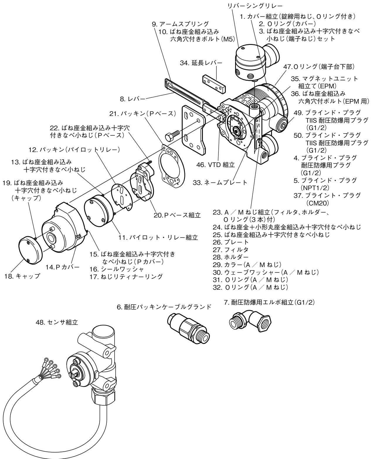
図 5-4 再販部品
