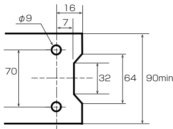
取付板参考図
