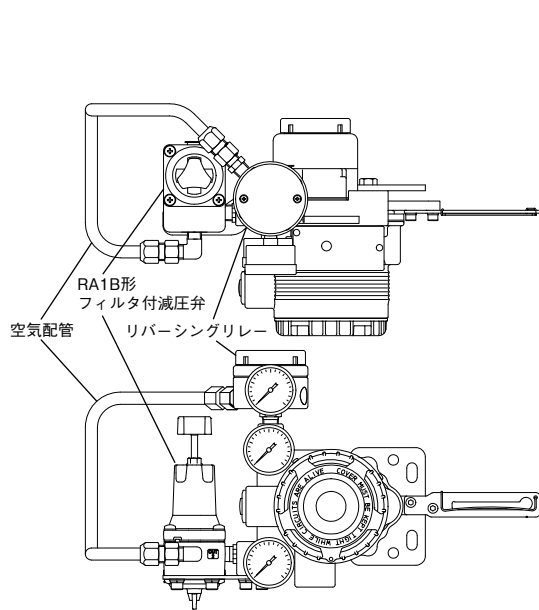
図 2-10-1 RA1B 組み付けのときの リバーシングリレーへの空気配管
