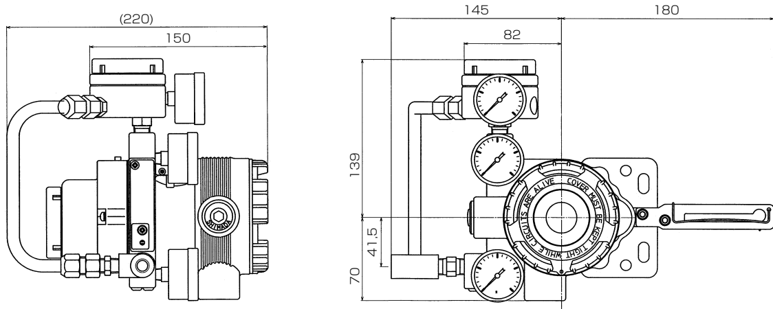
<複動用リバーシングリレー付、減圧弁なし>
