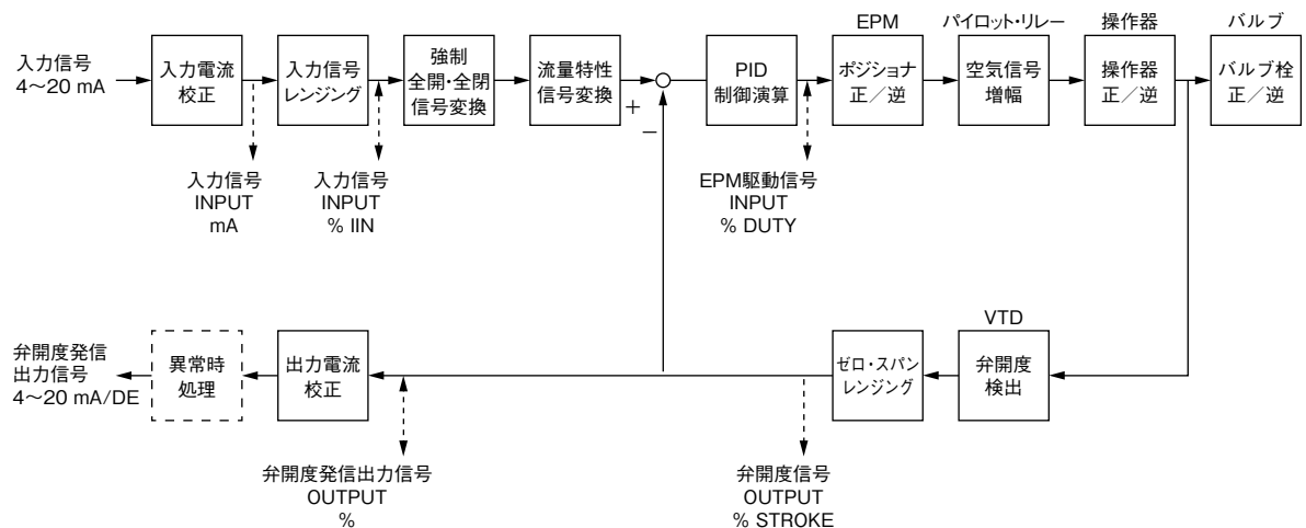
図 5-3 入出力フロー
