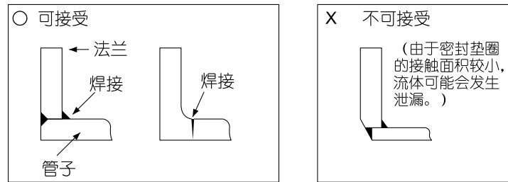
图 2-8 法兰形状
