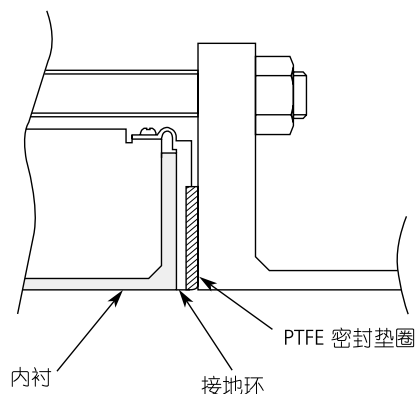
图 2-14 使用非不锈钢材质接地环和金属管道进行安装
