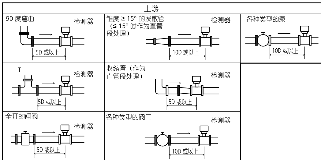
图 2-2 检测器上游侧的直管段 (D: 检测器公称内径)
