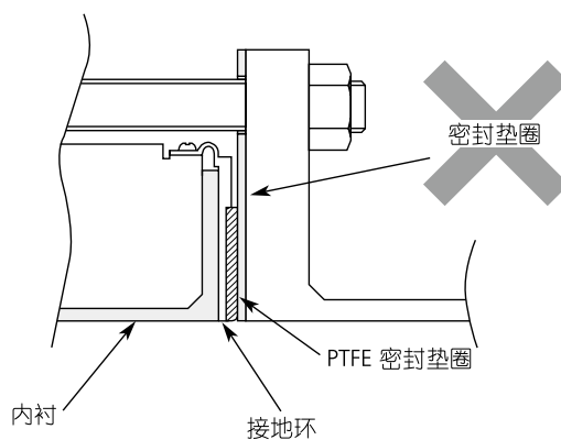
图 2-15 不正确的安装例
