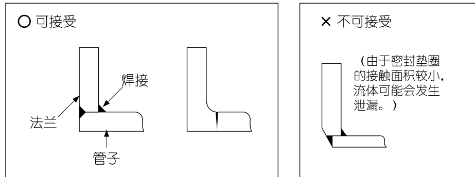
图 2-23 法兰形状
