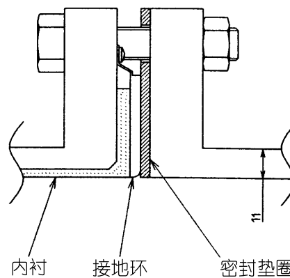
图 2-28 使用不锈钢材质接地环进行安装
