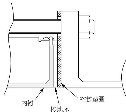
图 2-16 使用不锈钢材质接地环进行安装
