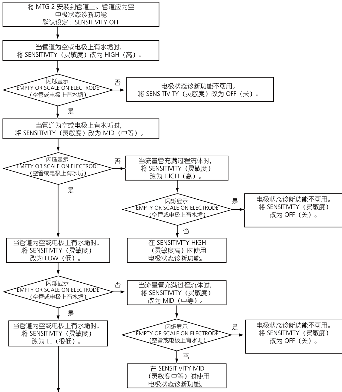
电极状态诊断流程图
