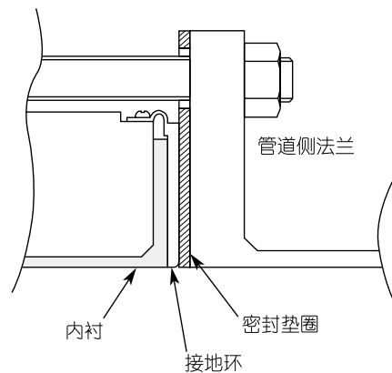
图 2-13 使用不锈钢材质接地环和金属管道进行安装
