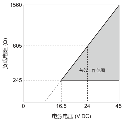
图 2-15. 电源电压和负载电阻特性
