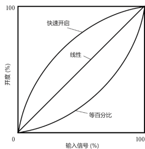
图 1. 输入-输出特性
