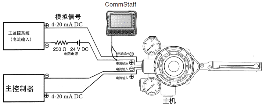
图 1-3. 模拟输出系统的结构（AVP301 型）
