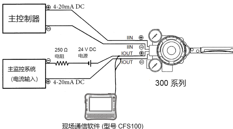
图 4-3 启用开度变送功能 (AVP301 型)
