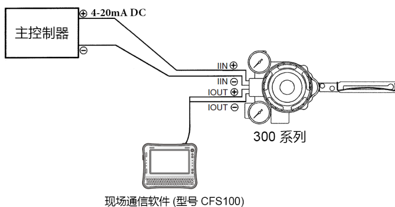
图 4-2 带现场通信软件 (型号 CFS100) (AVP300 型) 的配线
