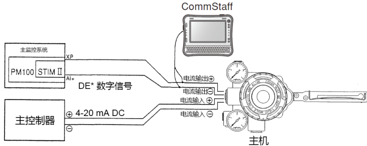
图 1-4. 数字输出系统的结构（AVP301 型）
