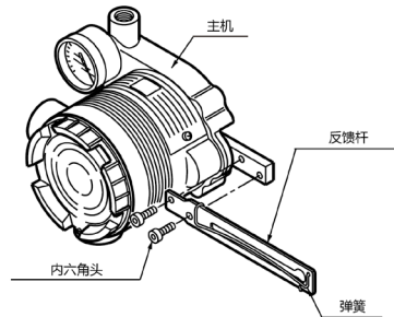
连接反馈杆
