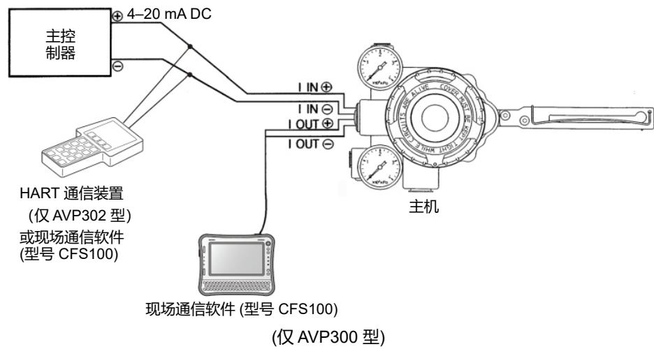
图 1-2. 无输出的系统结构 (型号 AVP300, AVP302)
