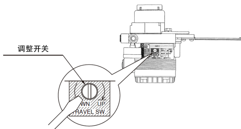
图 3-1 外部零点/满度调整装置的结构
