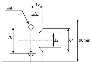
安装板参考图
