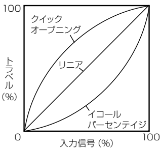
図4. 入出力特性
