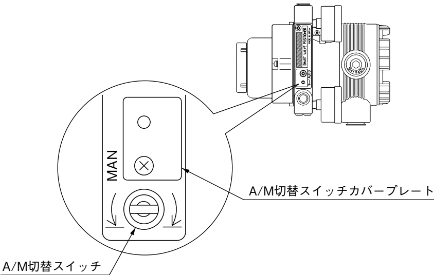
図5-1 A/M切替スイッチの構造
